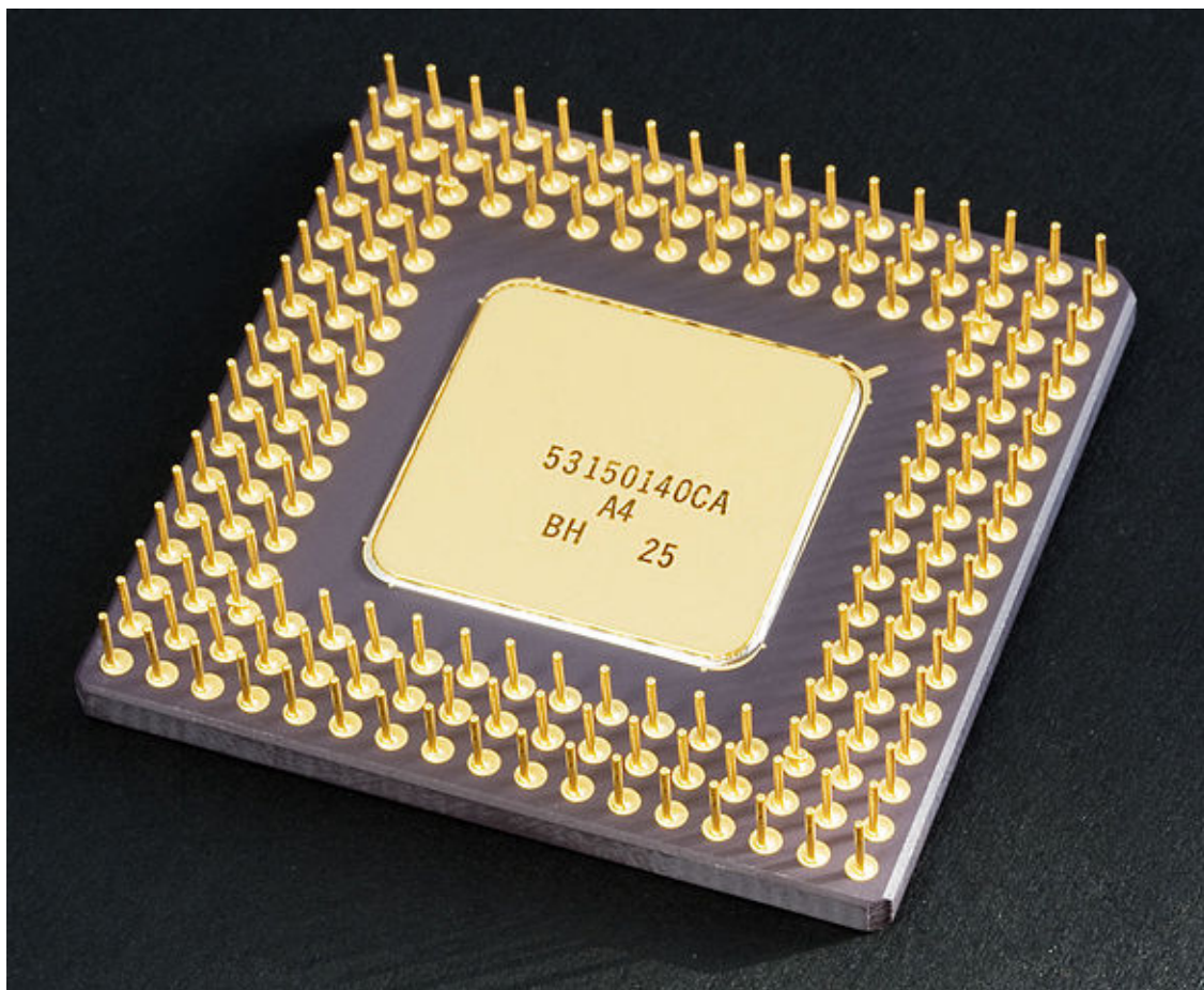
FIGURE II.1.1. – Arrière d'un processeur Intel 80486DX ( source ↗ )
