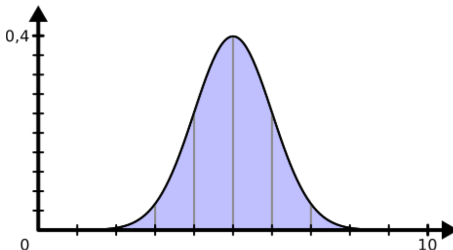
FIGURE VIII.2.3. – Densité de probabilité d'une distribution normale.
