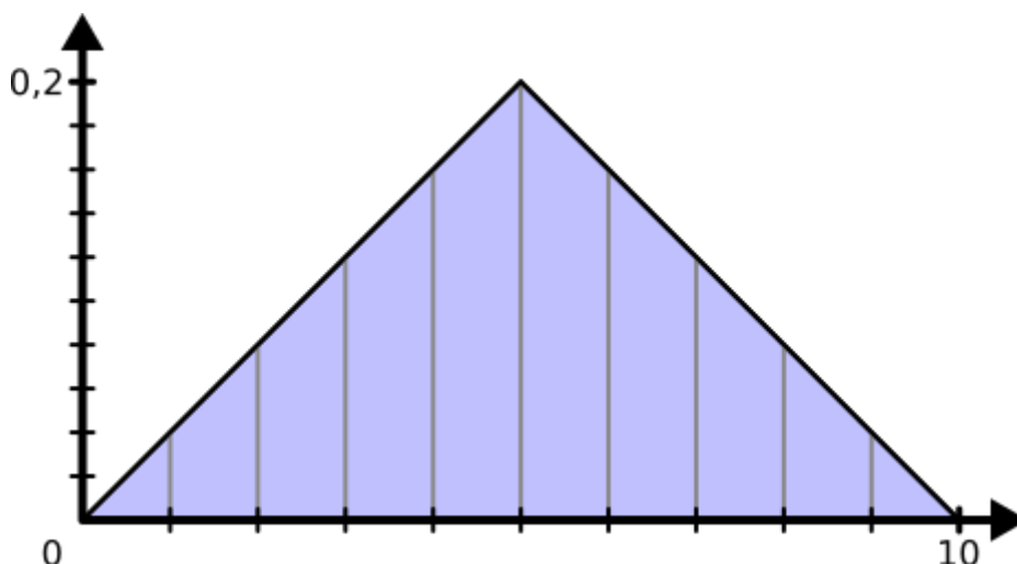
FIGURE VIII.2.2. – Densité de probabilité d’une distribution triangulaire.
