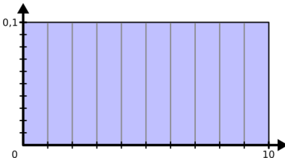
FIGURE VIII.2.1. – Densité de probabilité d’une distribution uniforme.
